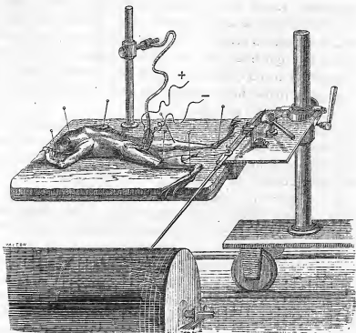
Fig. 3. — Myographe de Marey.
